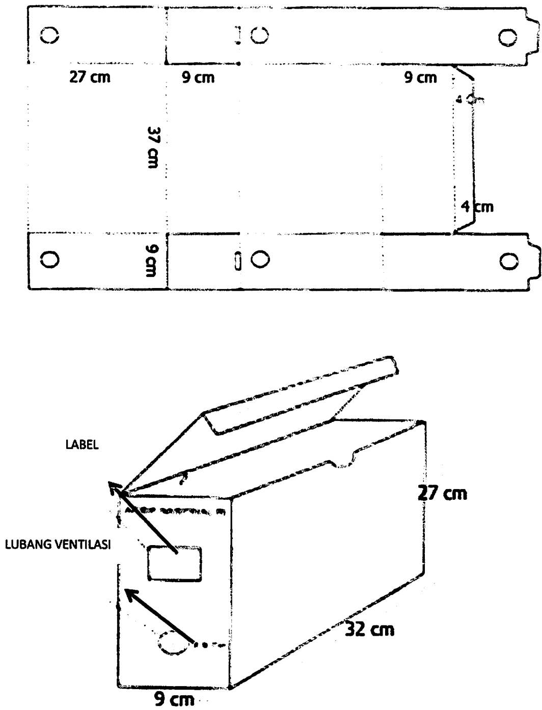
Gambar 2 Rancang Bangun Boks Arsip Kecil
